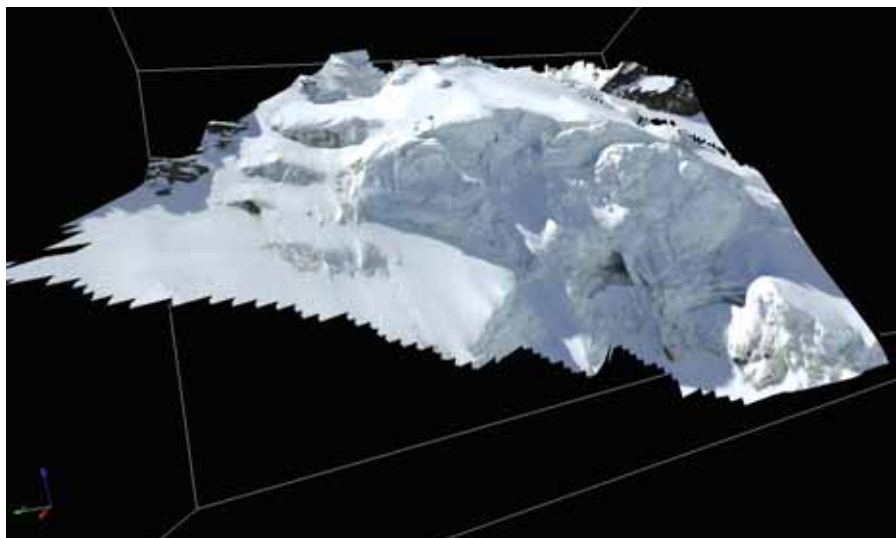
Il modello tridimensionale misurabile del terreno del seracco del San Matteo (Alta Valtellina) realizzato con il software JRC Reconstructor
